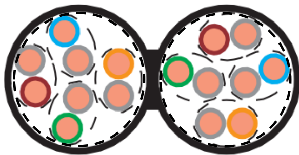
Abbildung 3: IT-Kabel der Kat.6 S/FTP Duplex (2x 4x2)
