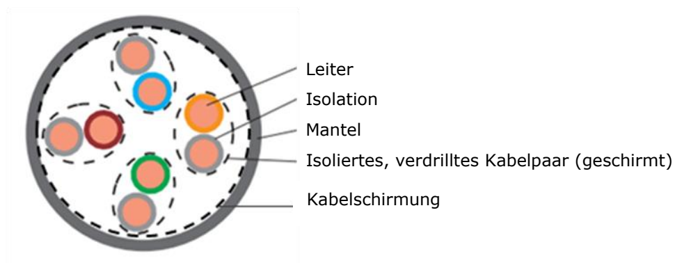
Abbildung 2: Netzwerk-Kabel S/FTP 4x2 zwischen MVT und Anschlussdose
