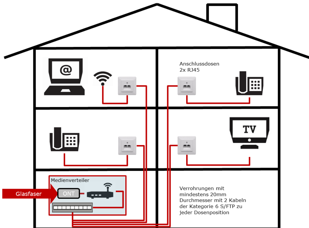
Abbildung 8: Interne Installation für Einfamilienhäuser mit der Installation des HAG im MVT
