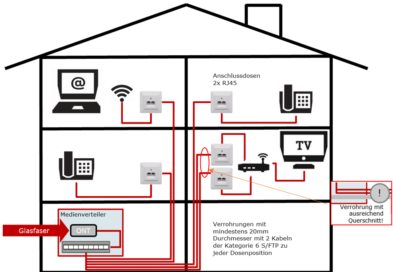
Abbildung 9: Interne Installation für Einfamilienhäuser mit HAG-Installation außerhalb des MVT
