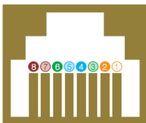
Abbildung 87: Kontaktbelegung Anschlussmodul RJ45
